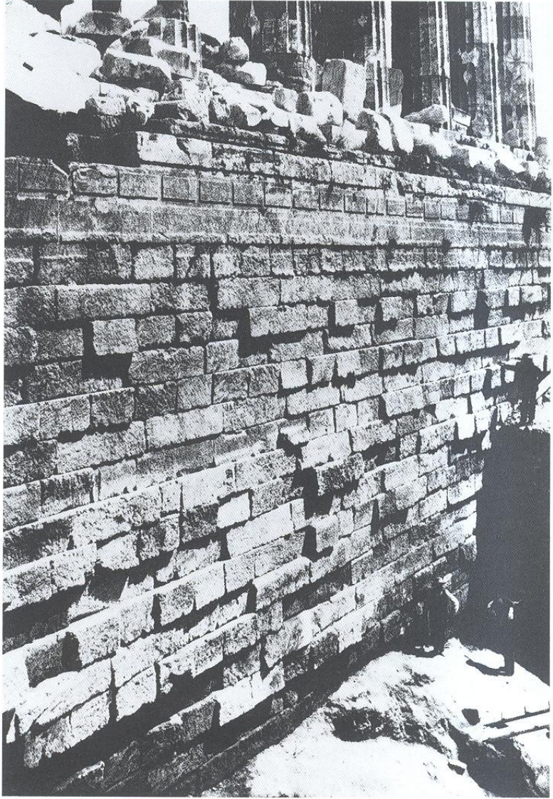
Το θεμέλιο του προπερίκλειου Παρθενώνος, όπως φαινόταν σε όλο του το ύψος τη διάρκεια των ανασκαφών του περασμένου αιώνα.
