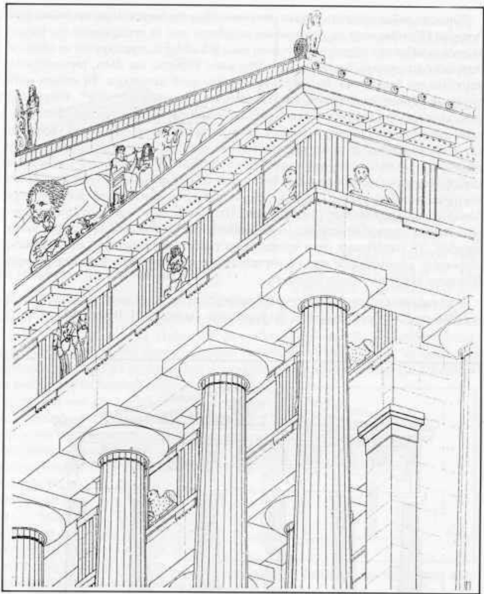
Εικ.19 Αναπαράσταση της ΒΑ γωνίας του "κτηρίου Η" (πρωταρχικός Παρθενών) Ο σήκος παρίσταται ως δίστυλος εν παραστάσιν, είναι, όμως, εξ ίσου πιθανόν ότι ήταν τετράστυλος πρόστυλος. Το γωνιαίο ακρωτήριο παρίσταται στην πρώτη, μετά την ανανέωση του βάθρου, μορφή. Το πρωταχικό ακρωτήριο (ή έλιξ) συνυπάρχει με το νέο. Το κορυφαίο ακρωτήριο παρίσταται ανανεωμένο για δεύτερη φορά (αλλαγή προγενεστέρου ανθεμίου ή γλυπτού και προσθήκη κορών εκστέρωθεν). Από την πρώτη ανανέωση παραμένει μόνον ο κεντρικός λίθος του βάθρου. Από το πρωταρχικό ακρωτήριο (Γοργώ) παραμένουν μόνον κατάλοιπα του μικρού υποβάθρου του κάτω από το πολύ μεγαλύτερο νέο βάθρον.
