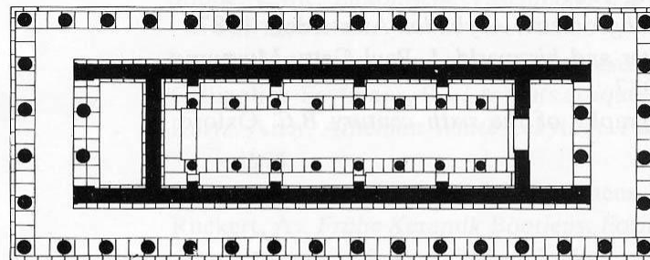
39. Κάτοψη αρχαϊκού Ηραίου Ολυμπίας. Γύρω στο 600 π.Χ.
