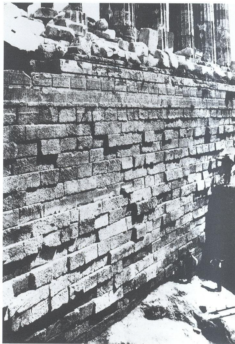
97. Το θεμέλιο του προπερίκλειου Παρθενώνας, όπως φαινόταν σε όλο του το ύψος πά τη διάρκεια των ανασκαφών του περασμένου αιώνα.
