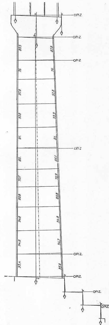
111. Σχῆμα τοποθέτησας τῶν σφονδύλων ἑνὸς κίονος εἰς τομὴν
