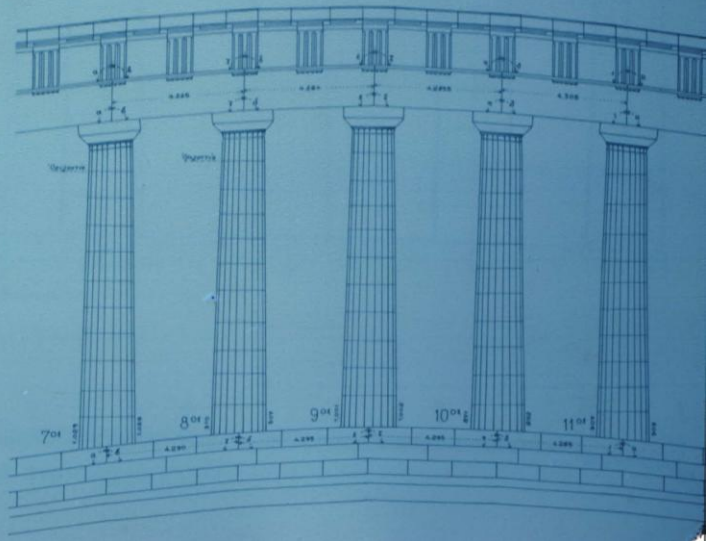
ΤΜΗΜΑ ΤΟΥ ΒΟΡΕΙΟΥ ΠΕΡΙΣΤΥΛΙΟΥ
