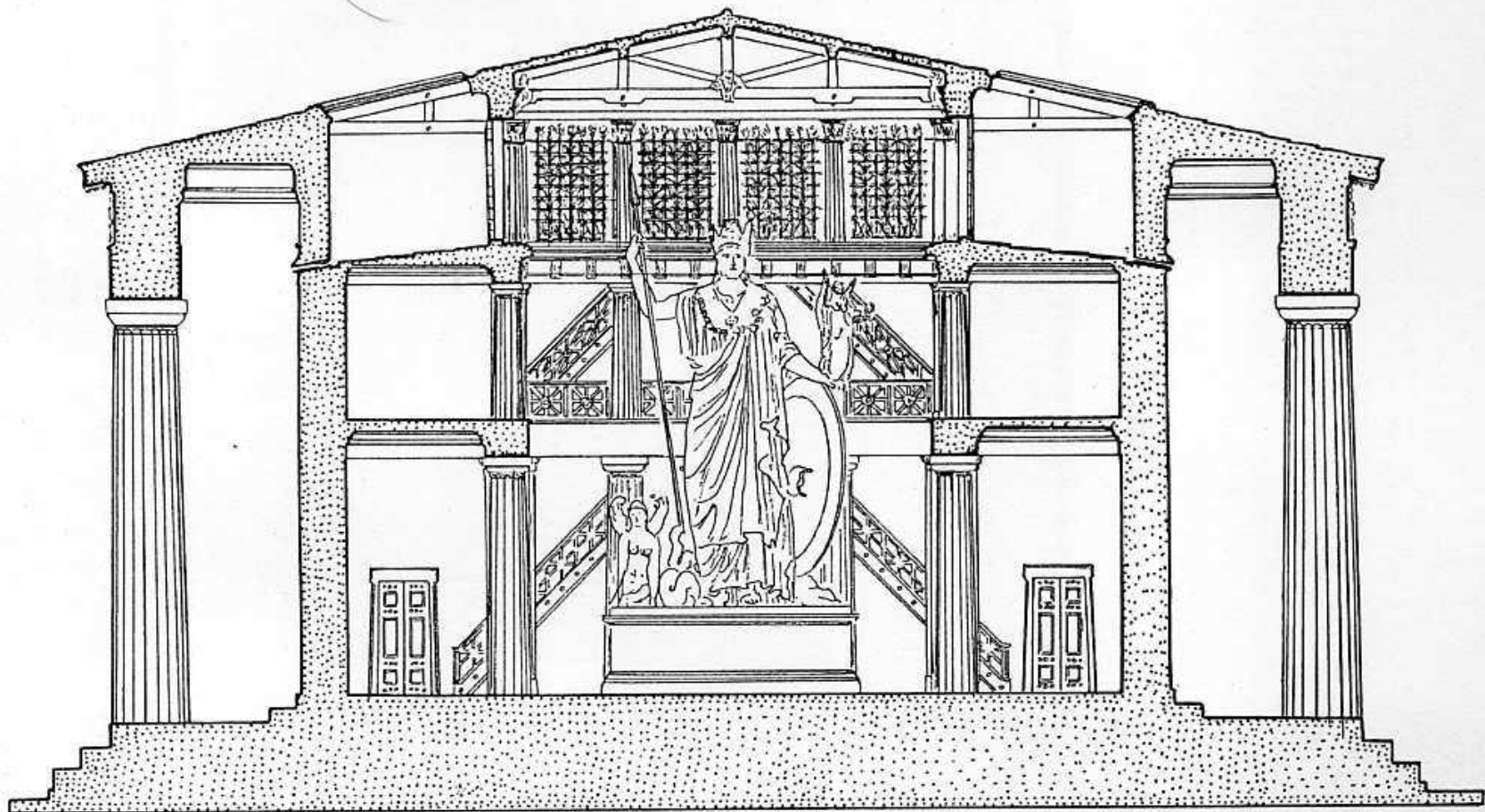
258. Προβολική αναπαράσταση εν κατά πλάτος τομή του εσωτερικού του κυρίου ναού του Παρθενώνος μετά φωταγωγού και διρρικού στέγης (κατά Fergusson).
