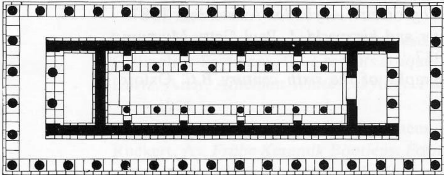
39. Κάτοψη αρχαϊκού Ηραίου Ολυμπίας. Γύρω στο 600 π.Χ.
