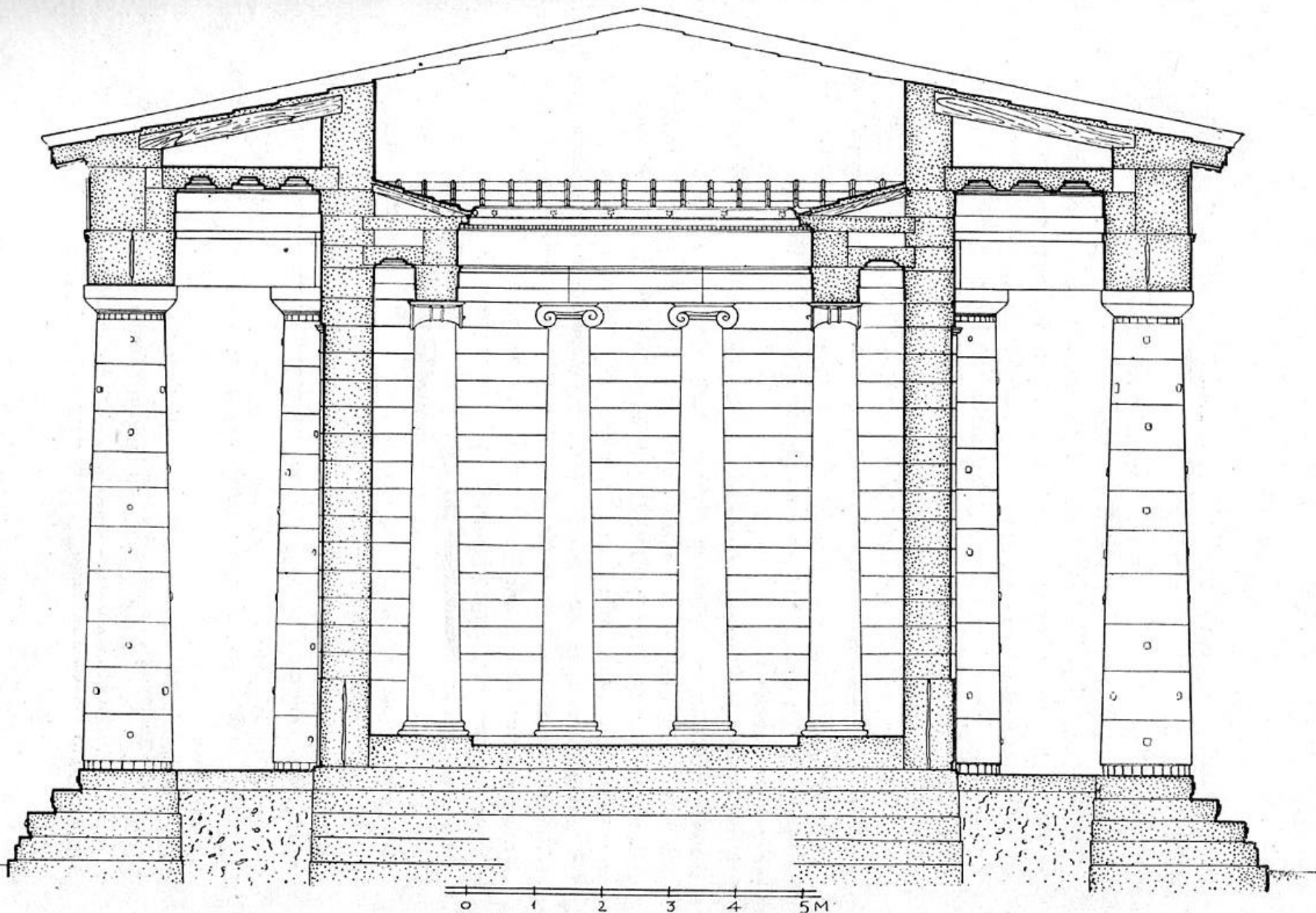
Εἰκ. 38. Τομή τοῦ ναοῦ κατὰ πλάτος (ἀναπαράστασις).
