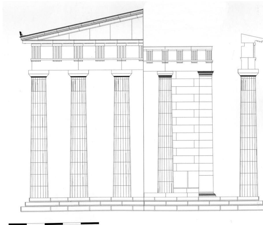
Ostansicht und Schnitt durch das Frontpteron, Ansicht der Pronaosfront – Rekonstruktion (M. 1 : 75)
