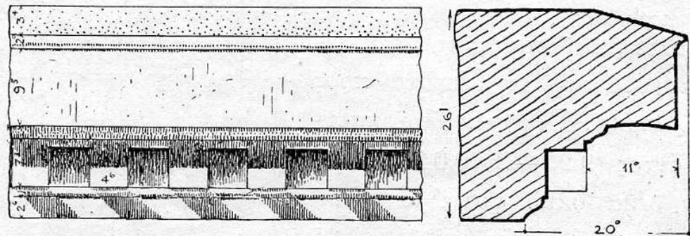
Εἰκ. 36. Γεῖσον τοῦ σηκοῦ. Πρόσοψις καὶ τομή.
