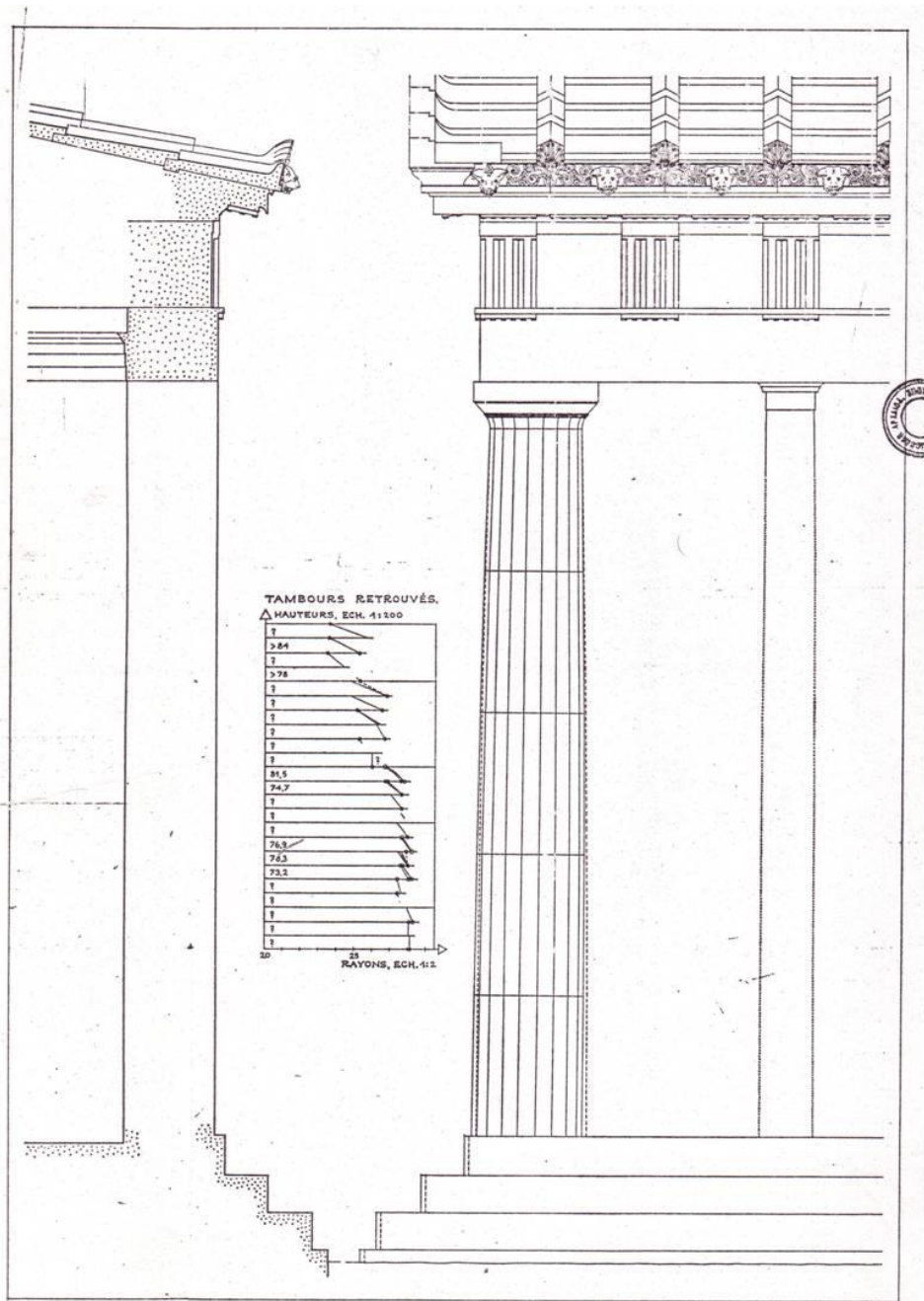
Ephèse. Temple d'Artemis. Elevation de l'ordre et coupe sur le mur du sécos (E. Hansen. Echelle 1:50).
