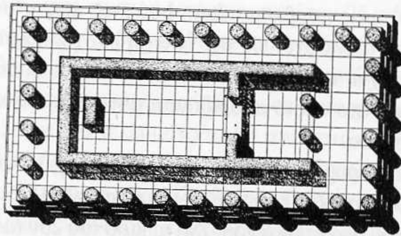
338. Κως, Ασκληπιείο. Δωρικός ναός του Ασκληπιού. Κάτοψη σε αναπαράσταση (1:600).
