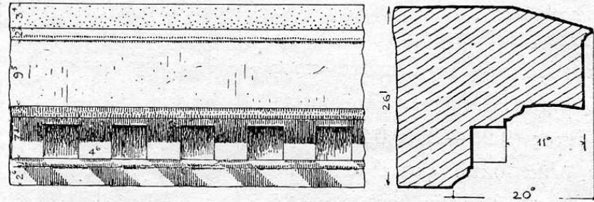
Εἰκ. 36. Γεῖσον τοῦ σηκοῦ. Πρόσοψις καὶ τομή.
