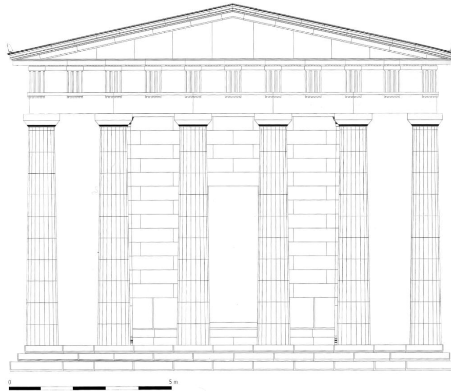
Ostansicht des Asklepios-Tempels – Rekonstruktion (M. 1 : 75)
