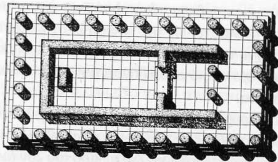
337. Κως, Ασκληπιείο. Δωρικός ναός του Ασκληπιού και στοές του ανώτερου ανδῆρου (1:400).
