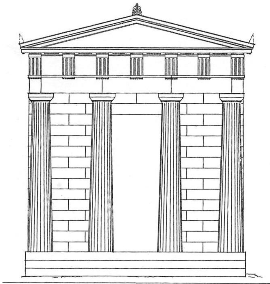
Fig. IV, 28. Reconstitution de la face nord du Temple.
