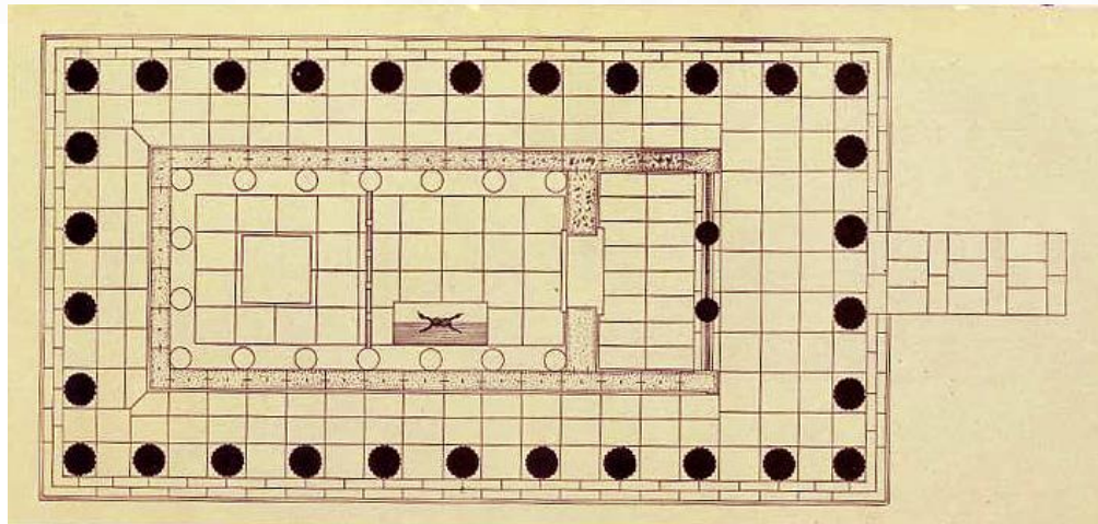
338. Κως, Ασκληπιείο. Δωρικός ναός του Ασκληπιού. Κάτοψη σε αναπαράσταση (1:600).
