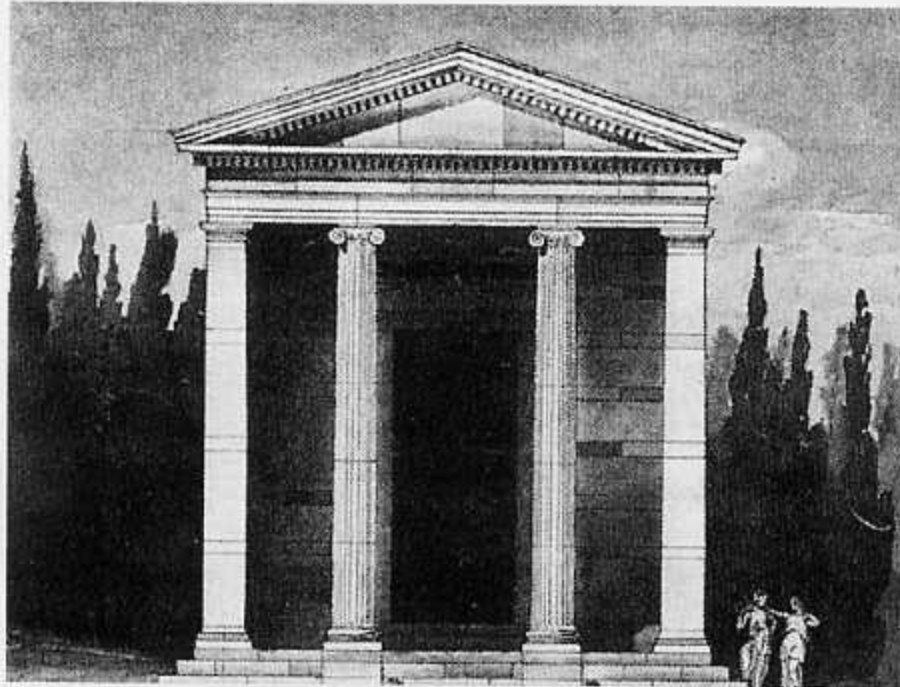
334. Κως, Ασκληπιείο. Ιωνικός ναός του Ασκληπιού (1:200).
