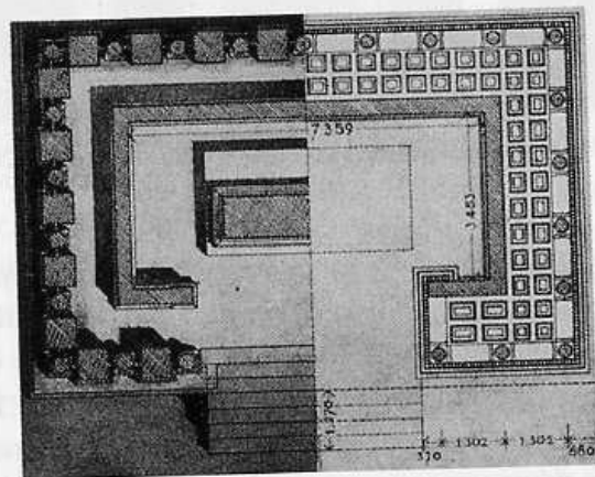
335/336. Κως, Ασκληρτείο. Ο βωμός, πρόσοψη σε αναπαράσταση και κάτοψη (1:200).
