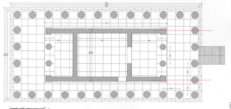
Rekonstruktion des Tempelgrundrisses (M. 1:125)
