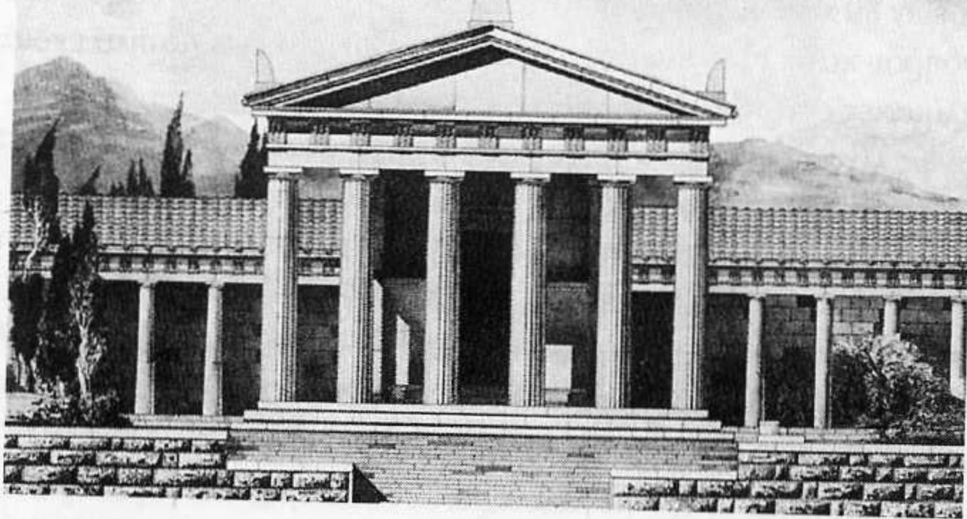
337. Κως, Ασκληπιείο. Δωρικός ναός του Ασκληπιού και στοές του ανώτερου ανδῆρου (1:400).
