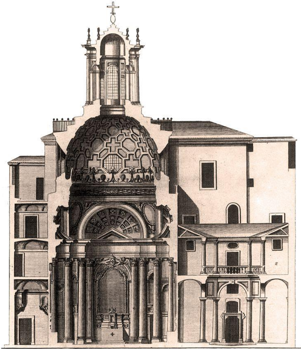
Francesco Borromini, San Carlo alle Quattro Fontane, 1637-41, Ρώμη. Τομή.
