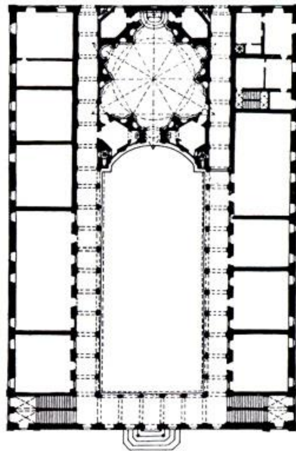
Francesco Borromini, Sant'Ivo alla Sapienza, 1642-1660, Ρώμη. Κάτοψη.
