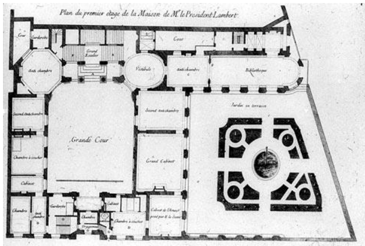
Louis Le Vau, Hôtel Lambert, 1640, Quai Anjou (Île Saint-Louis), Παρίσι. Κάτοψη.
