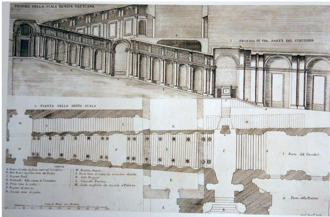
Gian Lorenzo Bernini, Scala Regia, 1663-66, Άγιος Πέτρος, Ρώμη. Τομή και κάτοψη.
