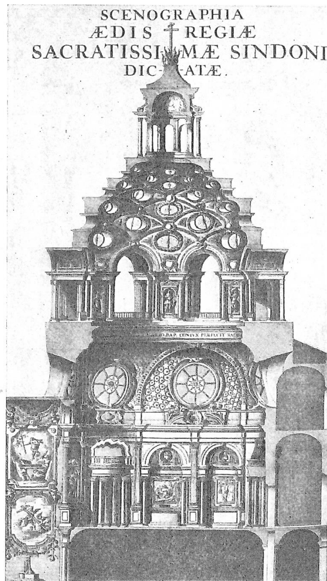
Guarino Guarini, Cappella della Sacra Sindone 1668–1694, Τορίνο, Ιταλία. Τομή.
