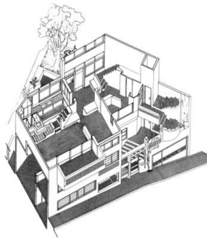
Δημήτρης και Σουζάνα Αντωνακάκη, Πολυκατοικία στην Εμμανουήλ Μπενάκη, Εμμανουήλ Μπενάκη 118, Αθήνα, 1972-75. Αξονομετρικό Σχέδιο.
