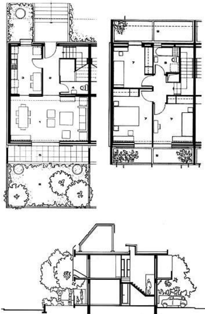
Γραφείο Μελετών Αλέξανδρου Ν. Τομπάζη Ε.Π.Ε, Ηλιακό Χωριό 3, Λυκόβρυση Αττικής, 1978-89. Κάτοψη (άνω) και τομή (κάτω) οικήματος.
