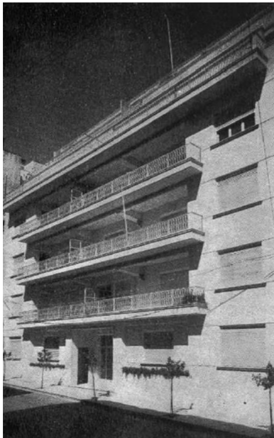
Ρέννος Κουτσούρης, Πολυκατοικία επί της οδού Σέκερη 4, Σέκερη 4, Αθήνα (1957). Γενική άποψη.
