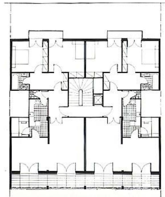
Νίκος Βαλσαμάκης, Πολυκατοικία Λούρου, Σεμιτέλου 5, Αθήνα, 1951-1953. Είσοδος πολυκατοικίας και τυπική κάτοψη ορόφου.
