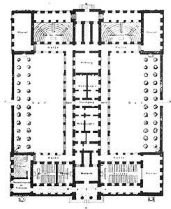
Hans Cristian Hansen, Εθνικό Καποδιστριακό Πανεπιστήμιο, Πανεπιστημίου 30, Αθήνα, 1839-1864. Κάτοψη.
