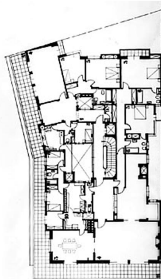
Εμμανουήλ Βουρέκα, Πολυκατοικία Αβέρωφ. Ηρώδου Αττικού και Μουρούζη, Αθήνα (1951). Κάτοψη ορόφου (ρετιρέ).
