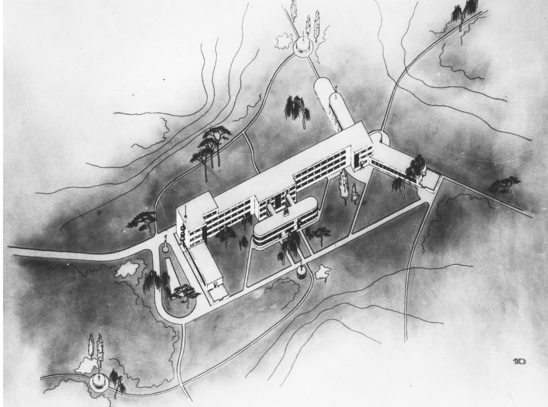
Ιωάννης Δεσποτόπουλος, Σανατόριο «Σωτηρία» (Περιφερειακό Γενικό Νοσοκομείο Νοσημάτων Θώρακος Αθηνών), Λεωφόρος Μεσογείων 152, 1932-37. Αξονομετρικό σχέδιο.
