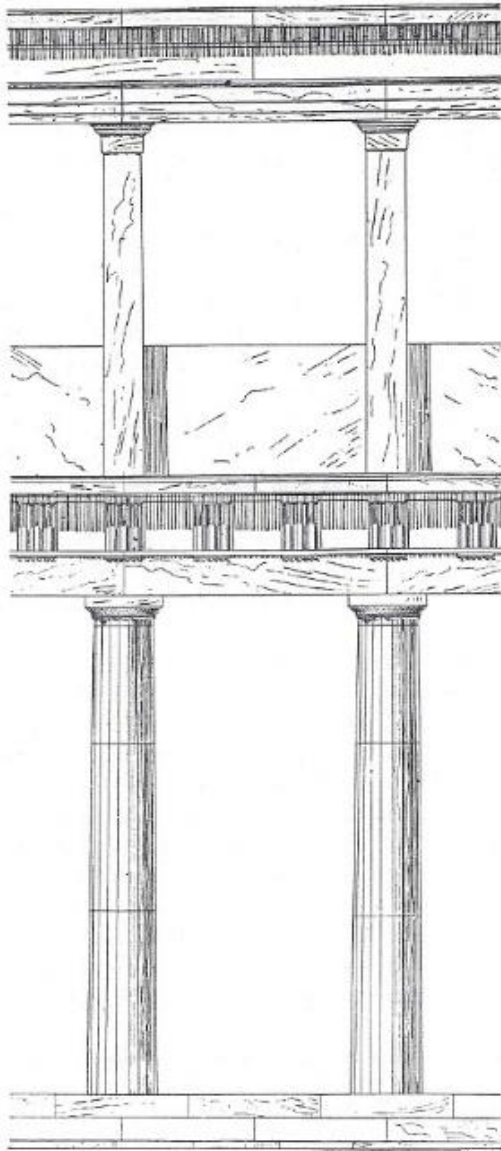
Fig. 1. — Délos. — Stoa coudée (détail). (Dessin de M. A. Gabriel.)
