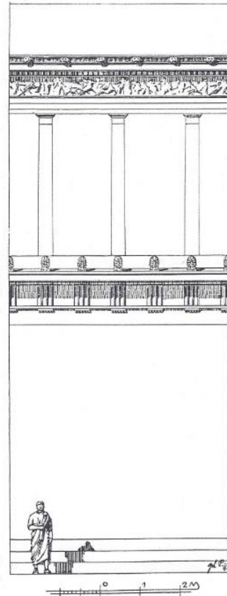
Fig. 3. — Délos. — Temple des Taureaux. Détail de la salle Nord. (Dessin de M. Gerh. Poulsen.)
