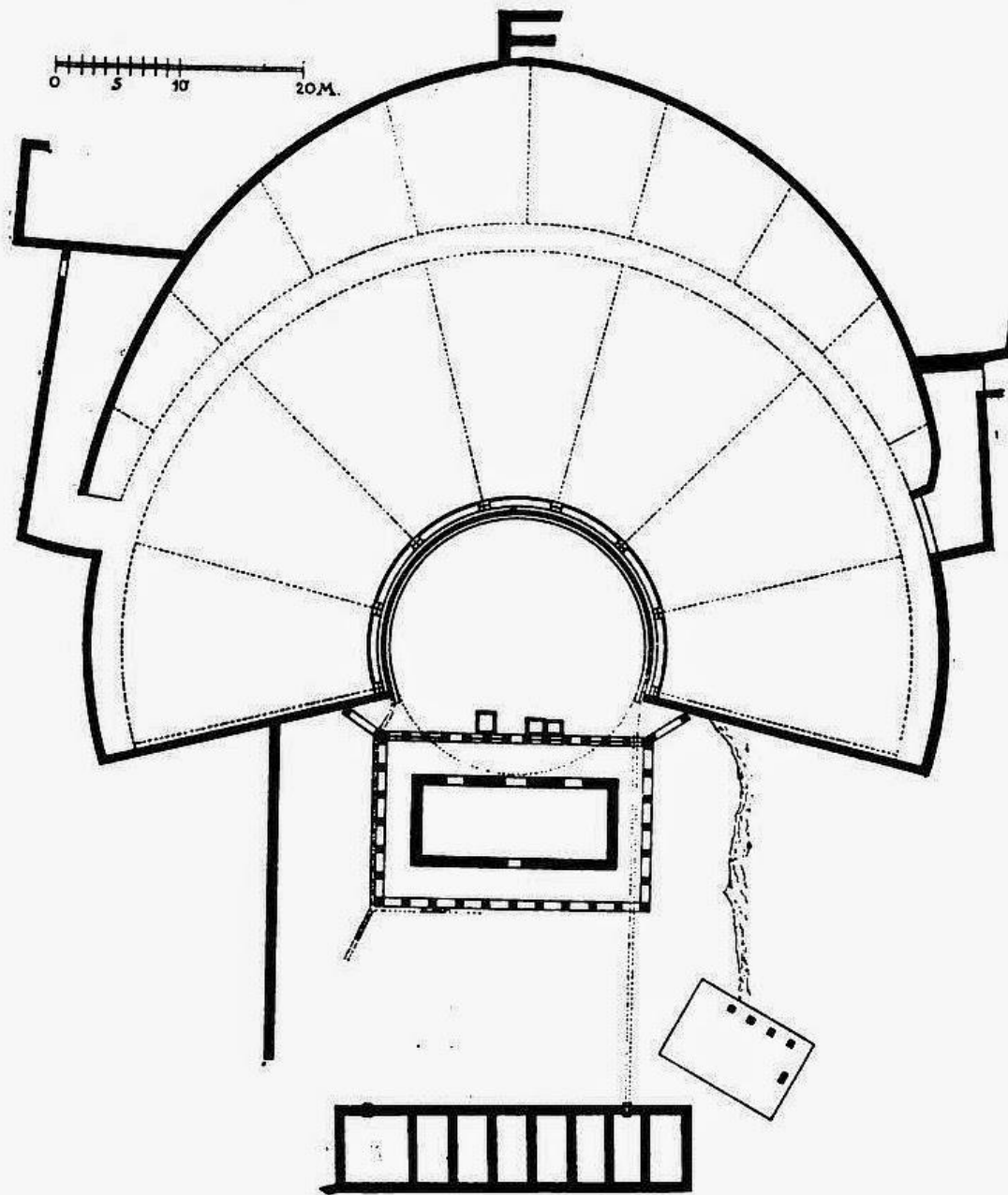
Figur 58. Grundriss des Theaters von Delos.
