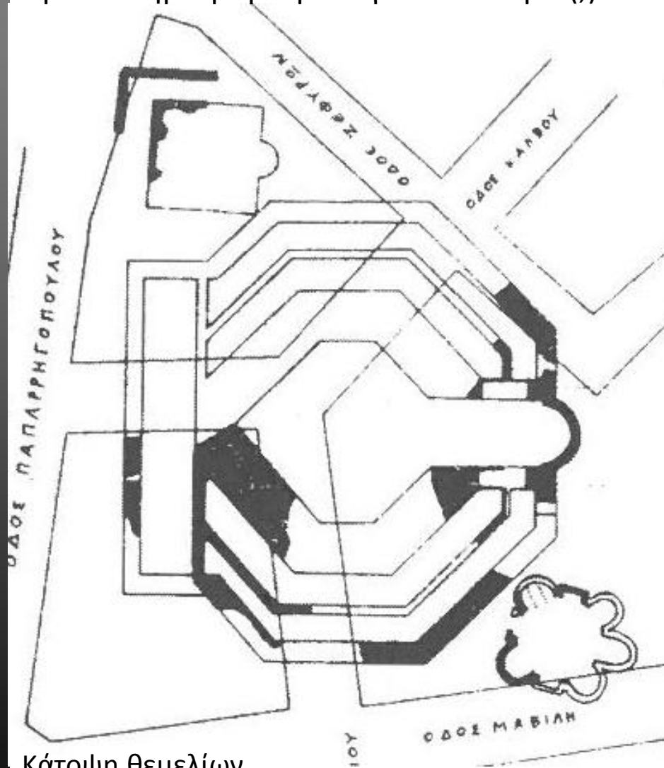
Κάτοψη θεμελίων
