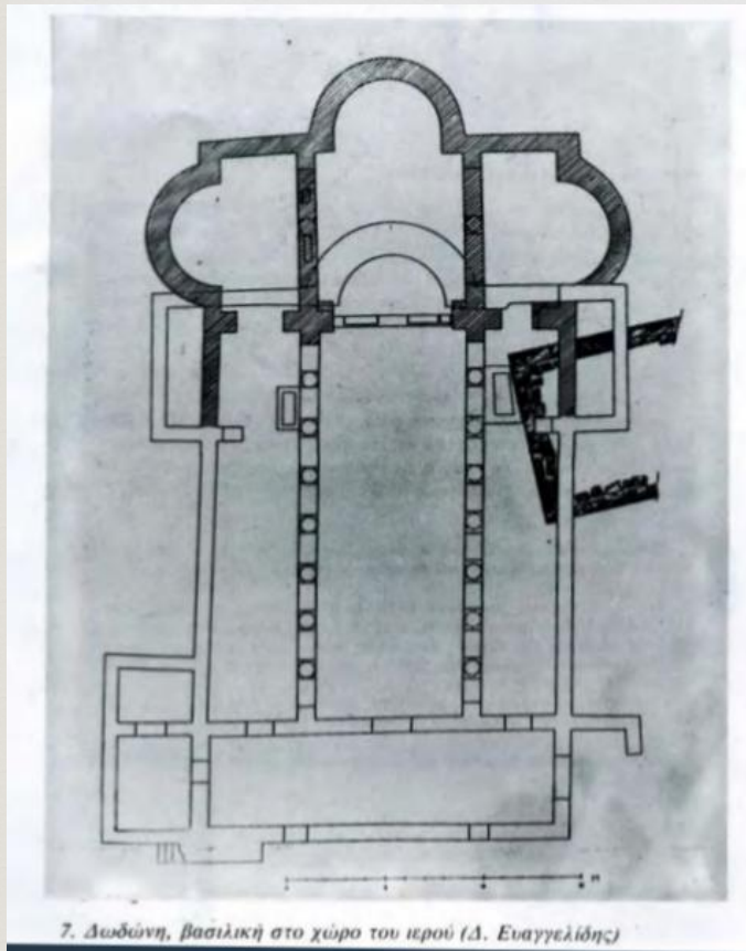
Κάτοψη Τρίκλιτης Βασιλικής Β', Ιερό Δωδώνης
