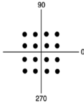
QAM-16
