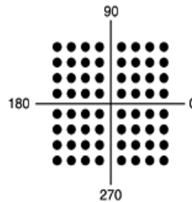
QAM-64
