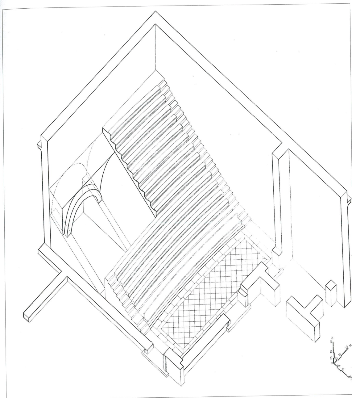
Fig. 5 - Ricostruzione assonometrica del cd. auditorium (da KNITHAKES-SYMBOLIDOU 1969)
