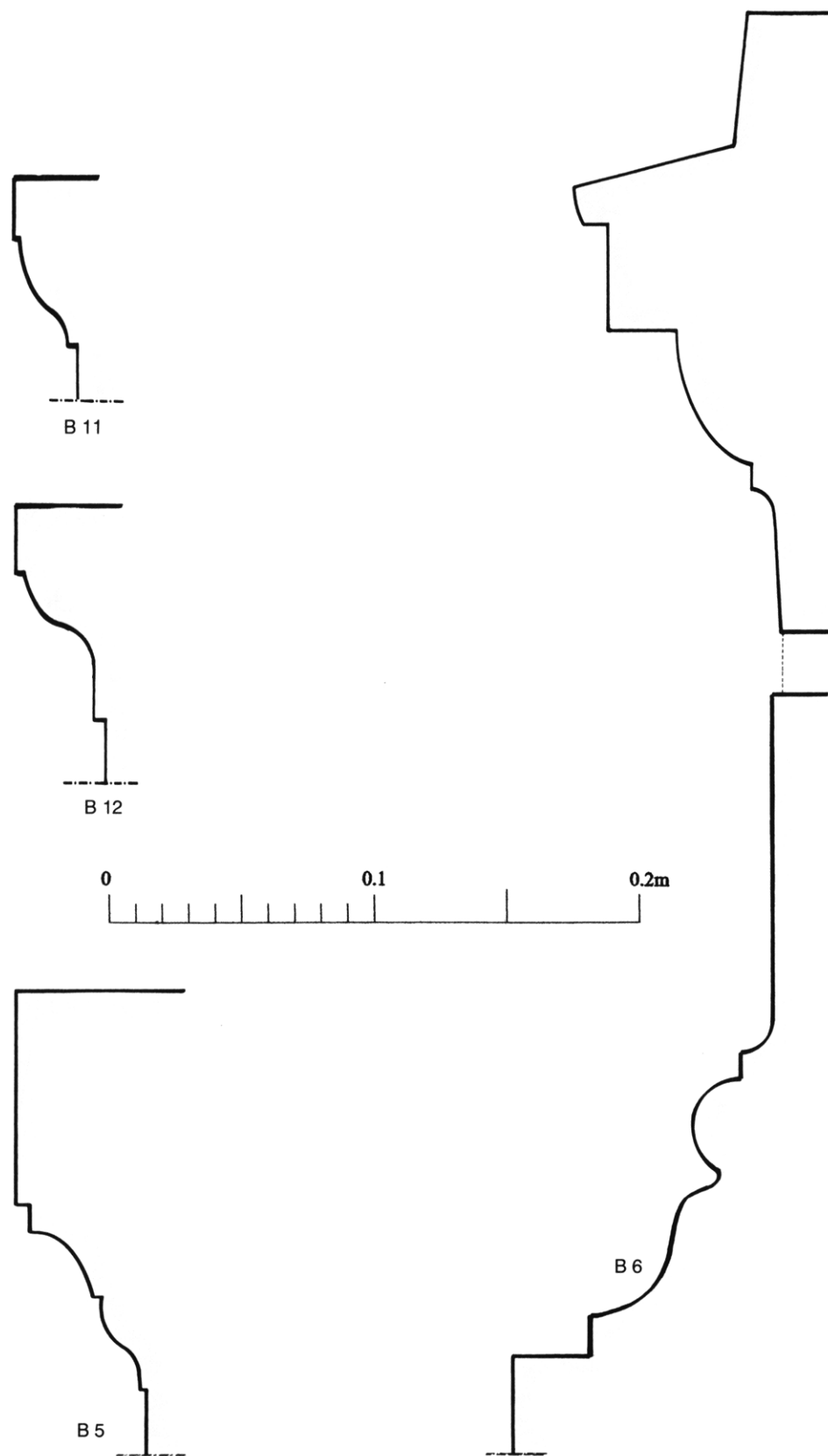
Εικ. 52. Κυμάτια βάθρων.
