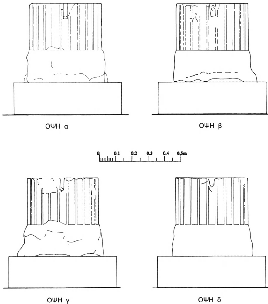
Εἰκ. 33. Κίονας Κ1, πλίνθος καὶ κάτω σφόνδυλος.
