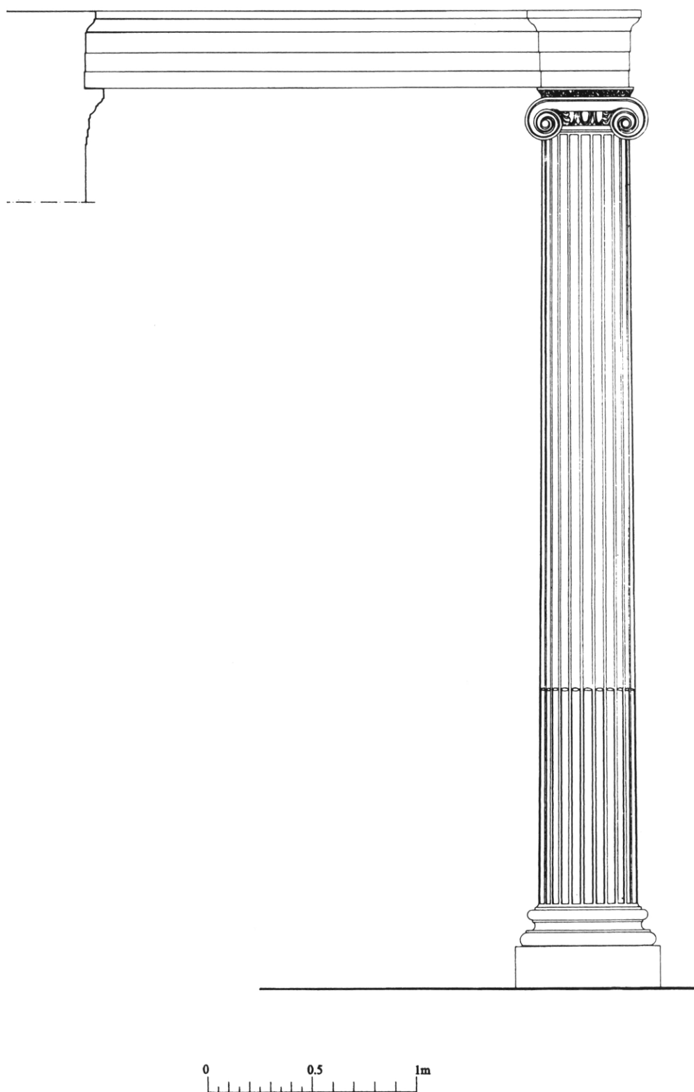
Εικ. 50. Ὁ ἰωνικὸς ρυθμὸς τοῦ Ἀρτεμίου, ἀναπαράσταση.
