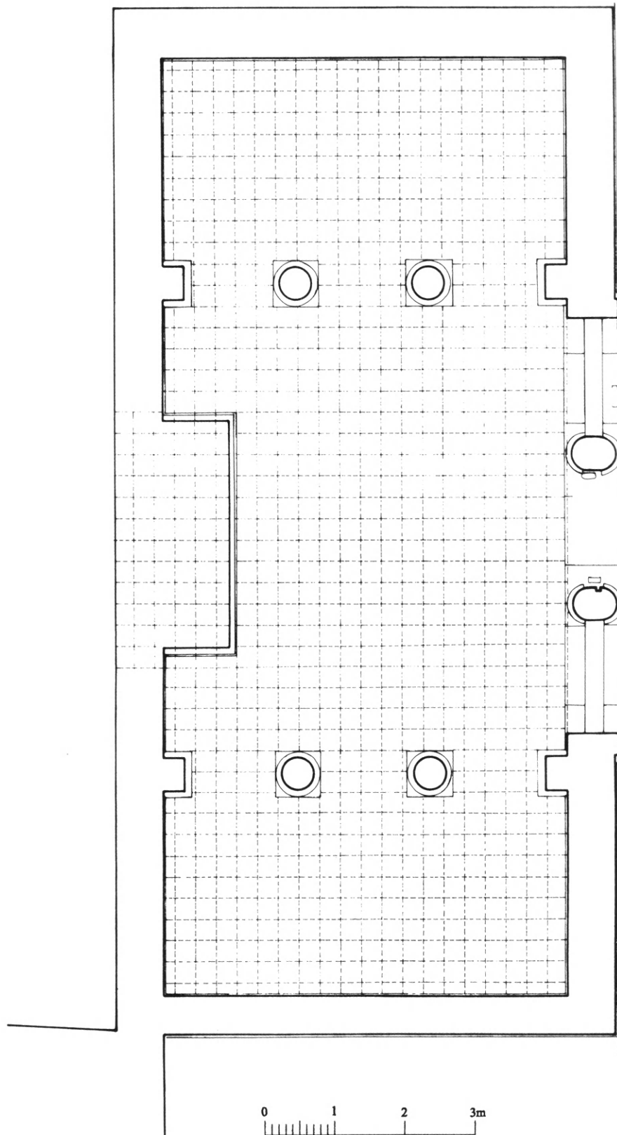
Εικ. 53. Έφαρμογή του κατασκευαστικού πόδα στην κάτωψη.
