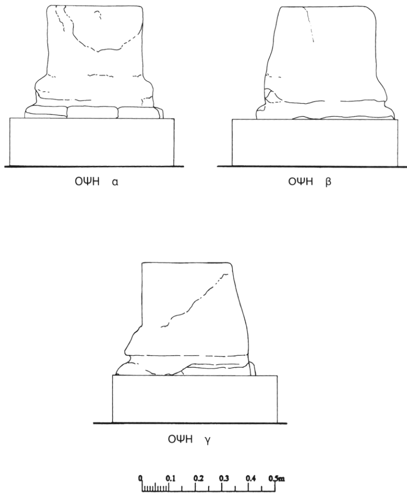
Εικ. 37. Κίονας Κ6, πλίνθος καὶ κάτω σφόνδυλος.
