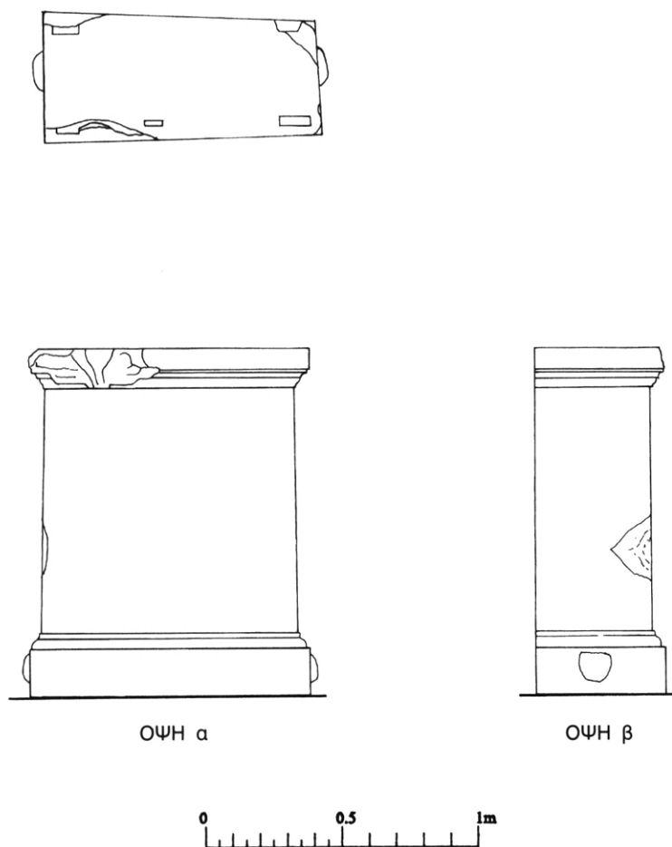
Εἰκ. 12. Βάθρο Β5.
