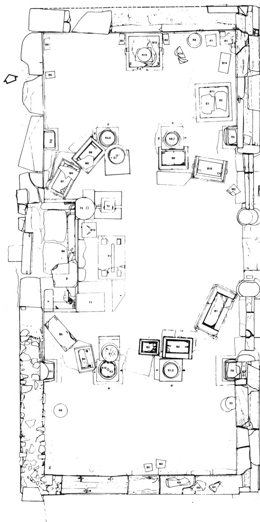
Εικ. 10. Κάτοψη του Ἀρτεμίου με ἀρίθμηση τῶν βάθρων καὶ τῶν ἀρχιτεκτονικῶν μελῶν.
