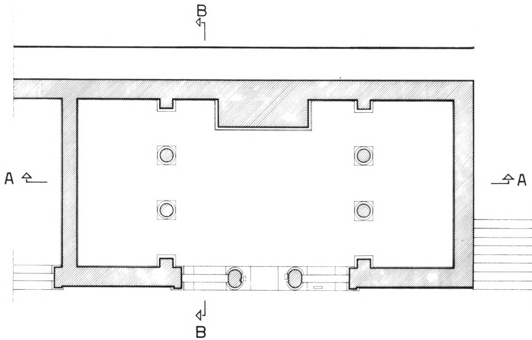
Εικ. 48. Αναπαράσταση της κάτοψης του Ἀρτεμείου.
