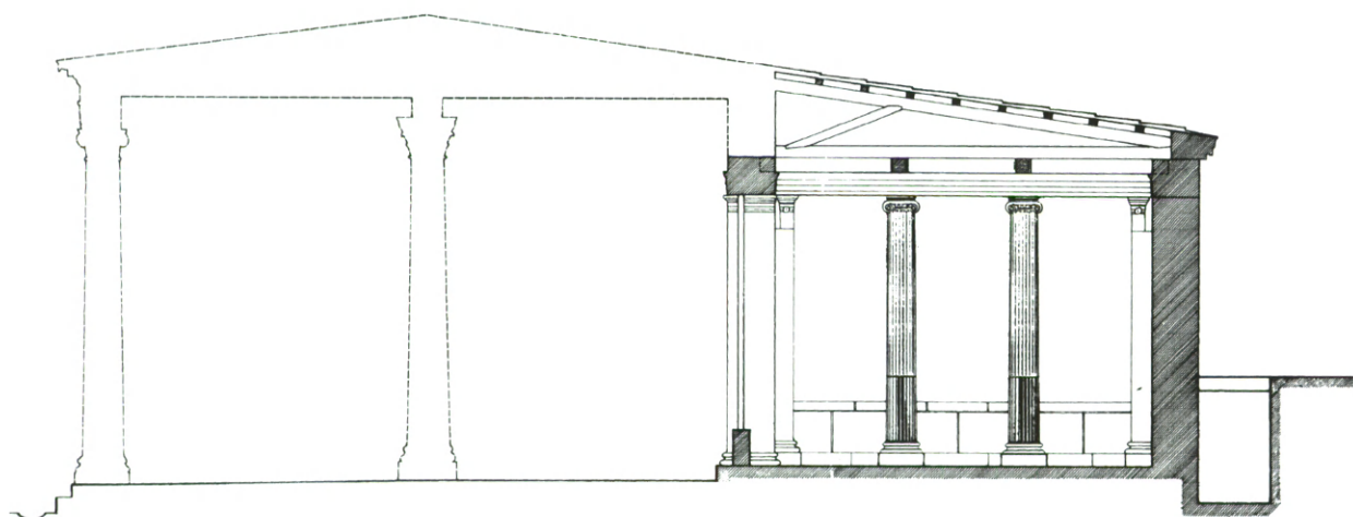
Εικ. 55β. Τομή ΒΒ με τη στοά, υπόθεση αναπαράστασης.
