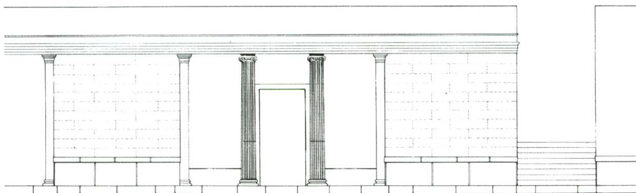
Εικ. 55α. Όψη στη στοά, υπόθεση αναπαράστασης.
