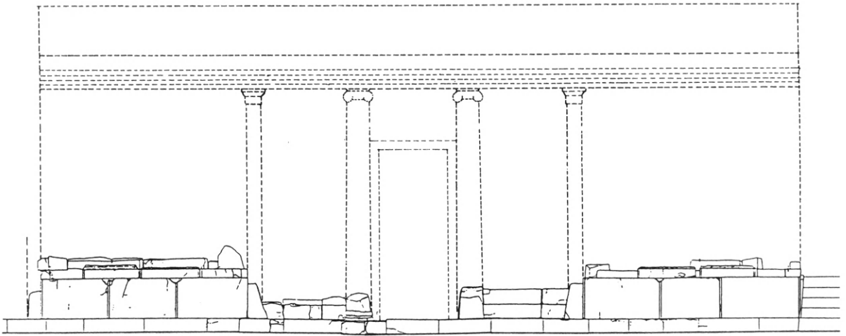
Εικ. 54α. Όψη στη στοά, υπάρχουσα κατάσταση και πρόταση αναπαράστασης.
