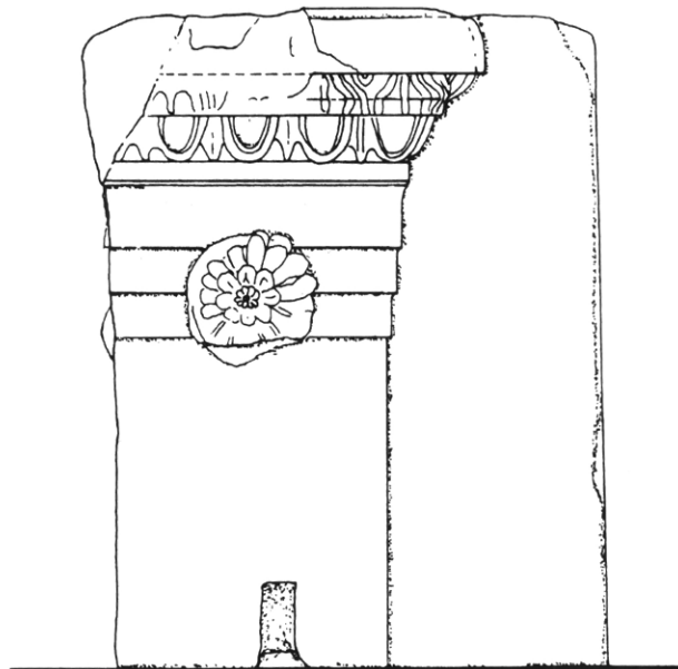
Εικ. 44. Ἐπίκρανο Ε1.
