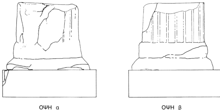
Εικ. 35. Κίονας Κ4, πλίνθος καὶ κάτω σφόνδυλος.
