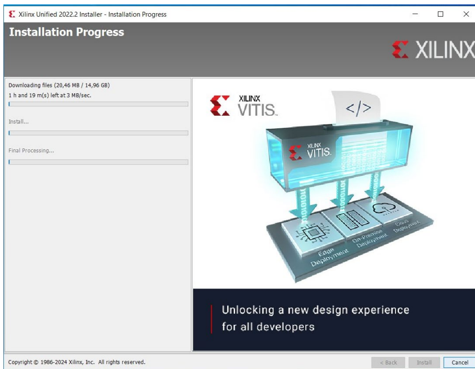
Εικόνα 19. Downloading Vivado
