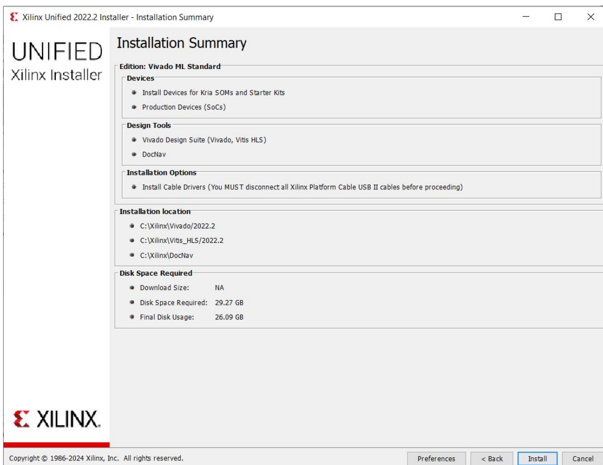
Εικόνα 27. Σύνοψη εγκατάστασης.
