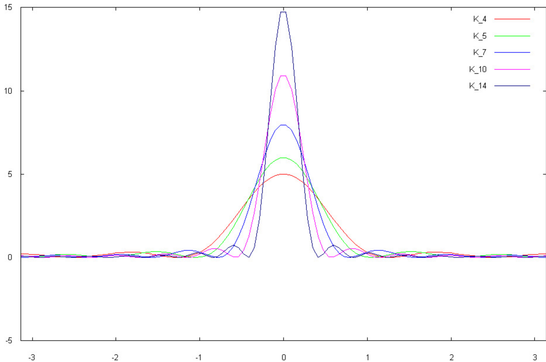
Ο πυρήνας του Fejer K_m για m=4,5,7, 10 και 14
