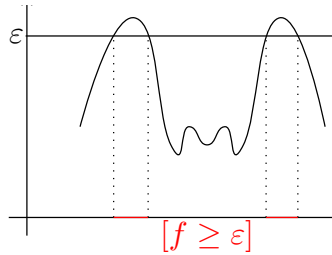
Σχήμα 7.1: Απόδειξη της ανισότητας Chebyshev-Markov
