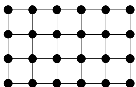
Σχήμα 1.7: H(6, 4) -σχάρα.
