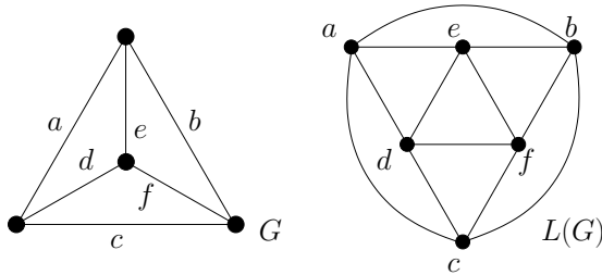
Σχήμα 2.1: Το γράφημα K_4 (τετράεδρο) και το γραμμικό του γράφημα L(K_4) (οκτάεδρο).
