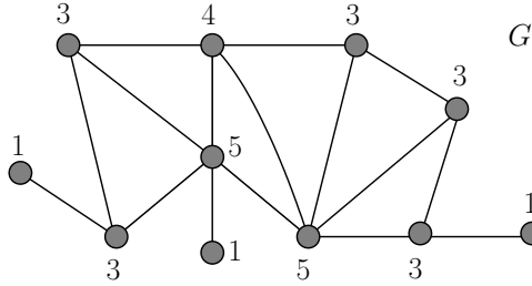
Σχήμα 3.3: Η γραφική ακολουθία που αντιστοιχεί στο γράφημα G είναι η [5, 5, 4, 3, 3, 3, 3, 3, 1, 1, 1] .
