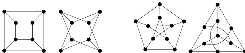
Το γράφημα του Petersen.
