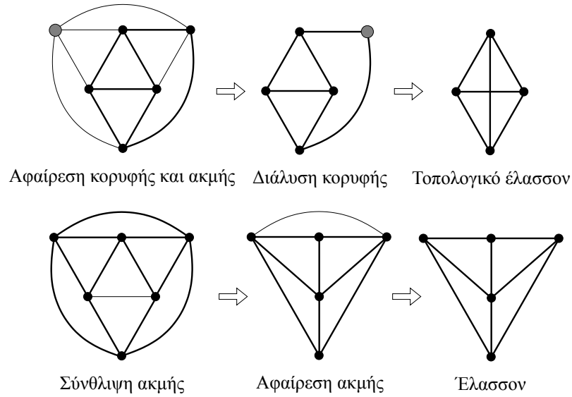
Σχήμα 2.7: Τοπολογικές σχέσεις
