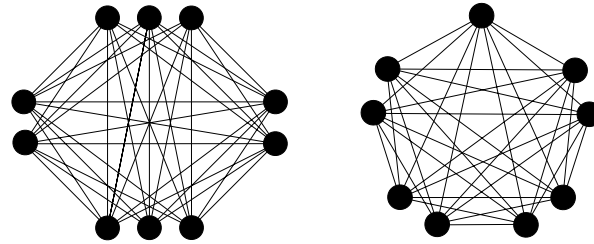
Σχήμα 9.2: Τα γραφήματα Turán T_4(10) και T_5(9) .
