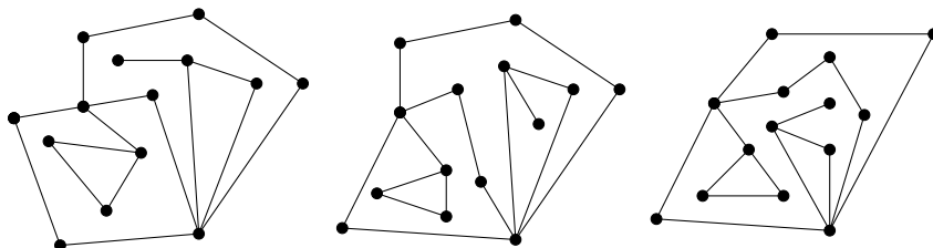
Σχήμα 7.2: Διαφορετικές εμβάπτισεις του ενεπίπεδου γραφήματος G_\Gamma όπου \Gamma το ενεπίπεδο γράφημα του Σχήματος 7.1.
