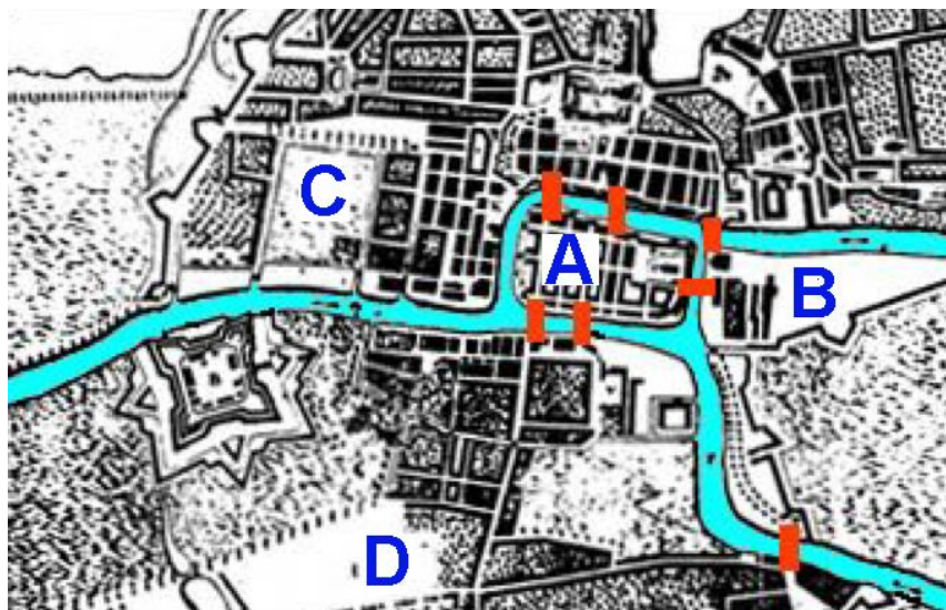
Σχήμα 12.2: Η πόλη Königsberg κατά τον 18 ο αιώνα και οι επτά γέφυρες πάνω από τον ποταμό Pregel. Το νησάκι στο κέντρο της πόλης στο οποίο προσπίπτουν 5 από τις 7 γέφυρες ονομάζεται Kniephof.
