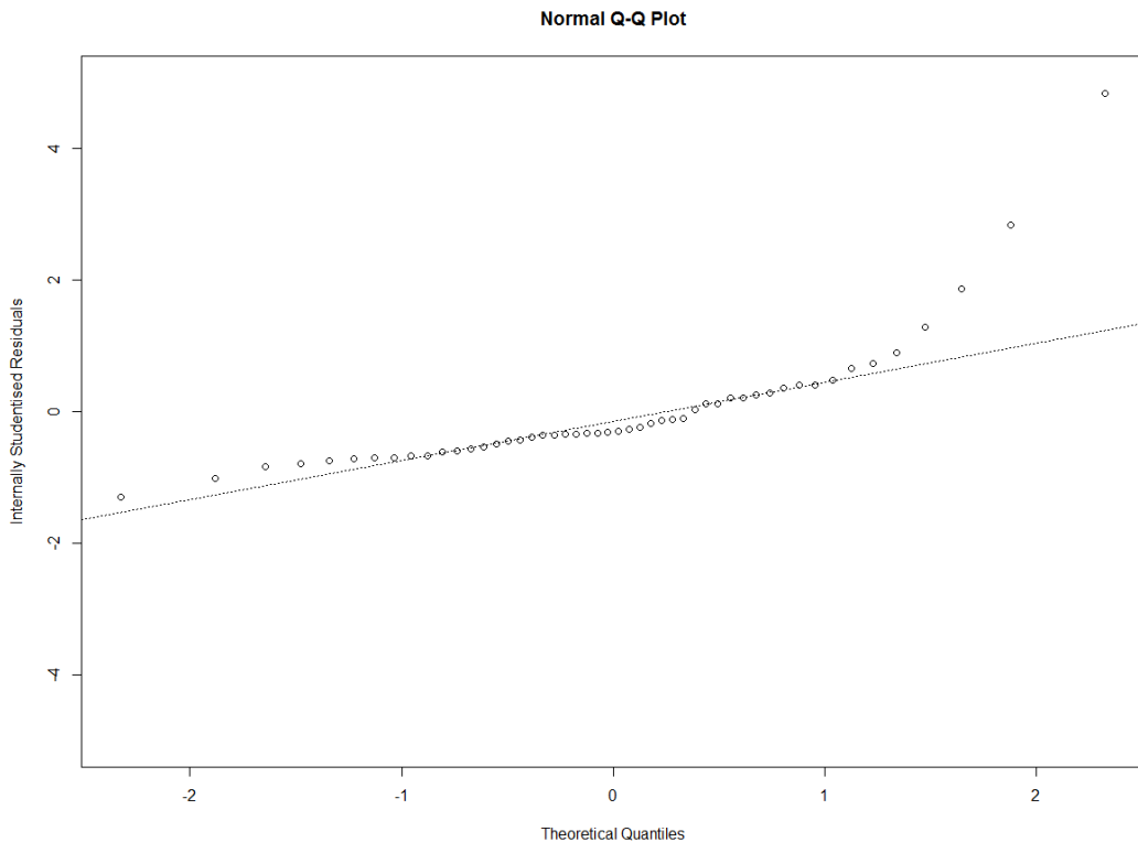
ΣΧΗΜΑ 2.7: Normal Q-Q Plot Μη-Κανονικά Κατανοημένων Καταλοίπων
