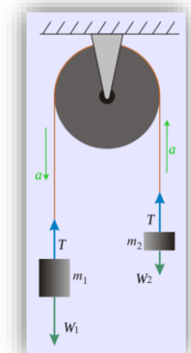
Μηχανή Atwood
