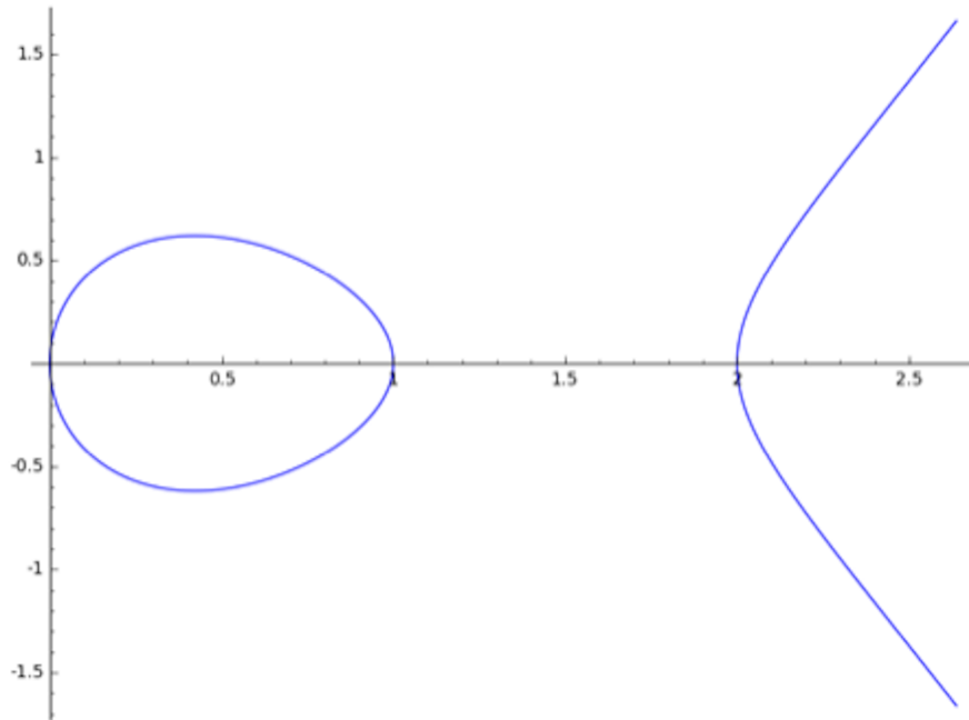
Σχήμα 7.4. Για \lambda = 2 έχουμε τη γραφική παράσταση:
