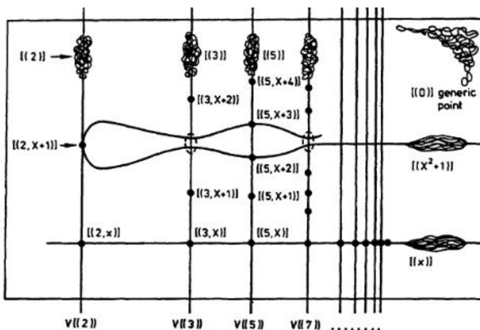
Σχήμα 2.5. Πρώτα ιδεώδη των πολυωνύμων με συντελεστές ακέραιους
