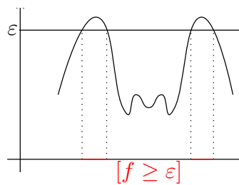
Σχήμα 6.2: Απόδειξη της ανισότητας Chebyshev-Markov
