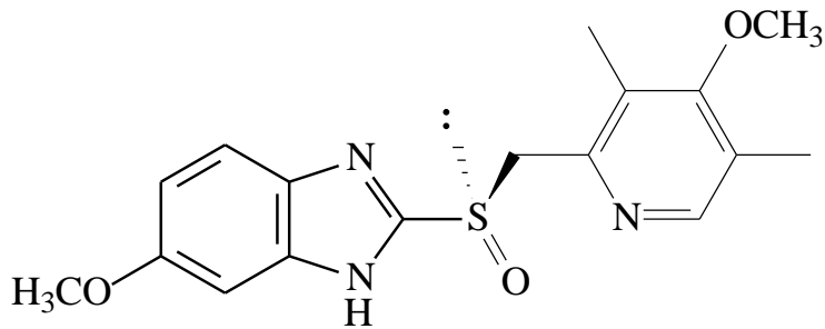
R -(+)-εναντιομερές
