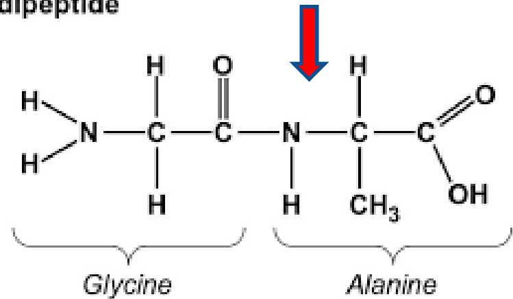
A dipeptide
