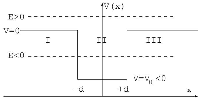
Σχήμα 1: Πηγάδι δυναμικού σε μία διάσταση.
