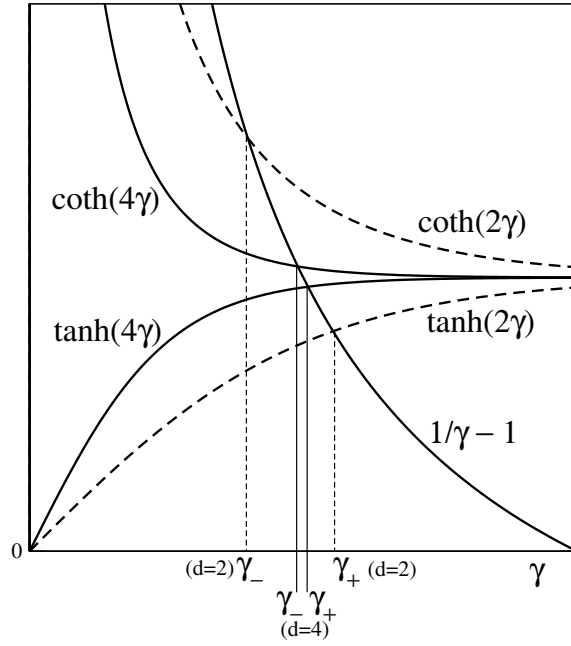
Σχήμα 5: Γραφική λύση των εξ. (175) για d = 2 και d = 4 .
