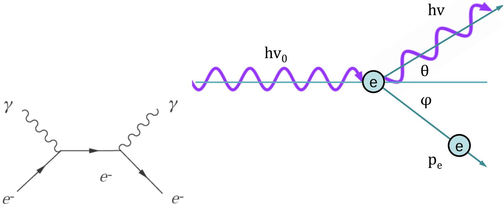
Διάγραμμα Feynman
