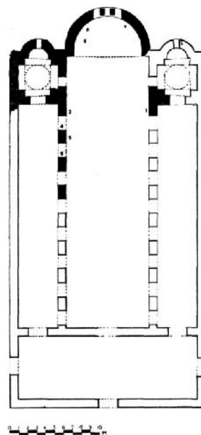
Εικ. 1. Κάτοψη της Βασιλικής του 'Αγ. 'Αγγελαίου.
