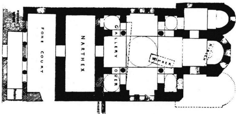
Τρίγλεια Βιθυνίας, Fatih Camii, αρχές 9ου αι. (κάτοψη).
