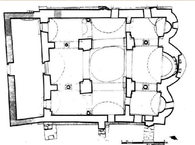
Πλησιοί Άρτας, Άγιος Δημήτριος του «Κατσούρη», π. 800 (κάτοψη).
