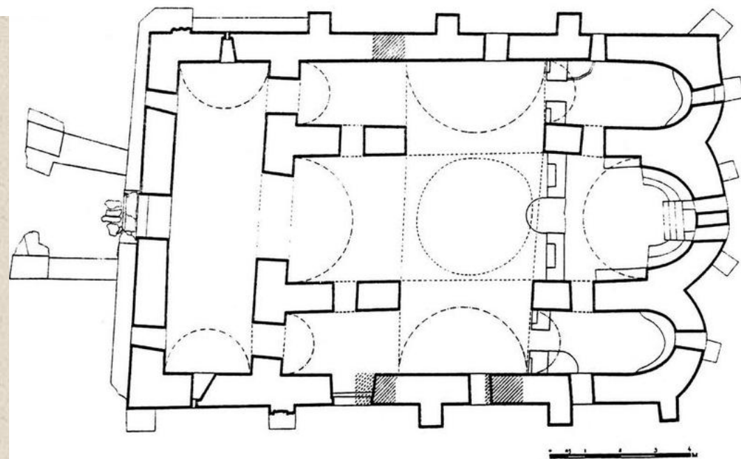
Εφρυτανία, Έπισκοπή, π. 800 (κάτοψη).
