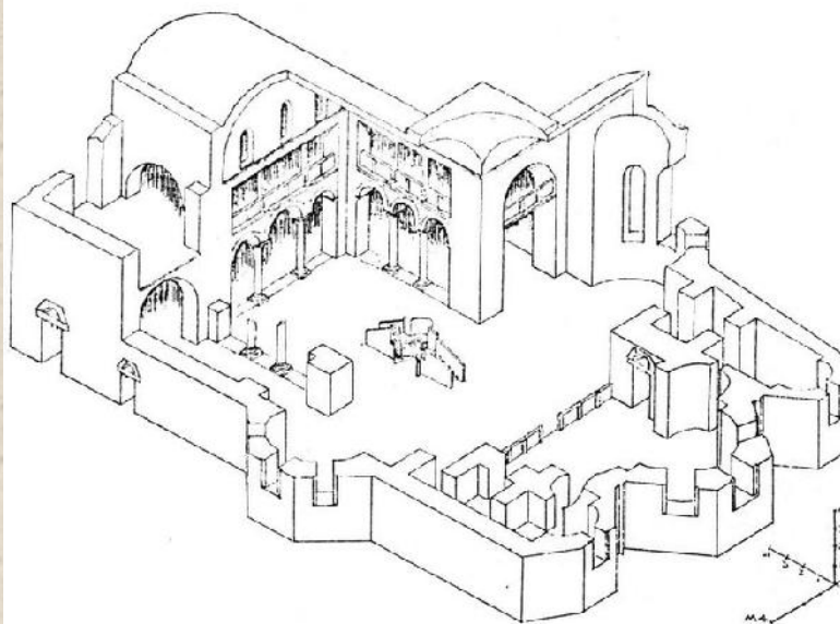
Κρήτη, Γόρτυνα, "Άγιος Τίτος, 7ος αι. (ισομετρική ἀποκατάσταση).
