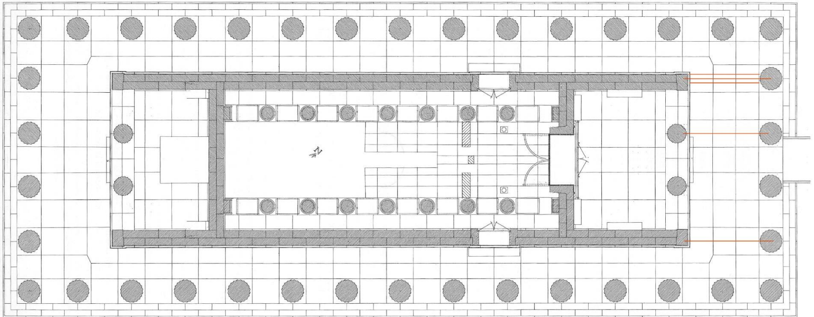
Fig. 18.19. Plan, Restitution éch. 1/225.
