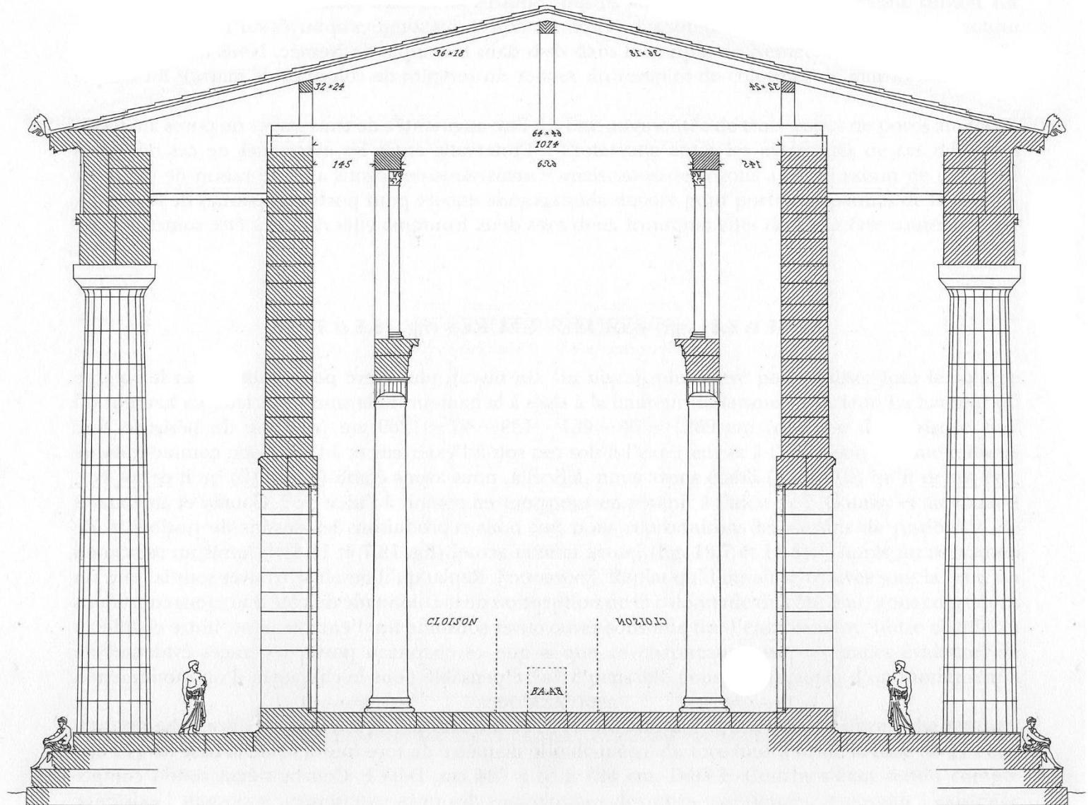
Fig. 18.5. Coupe sur la cella, avec les portes latérales. Essai de restitution éch. 1/125. Les détails des colonnades intérieures sont hypothétiques et la restitution de la charpente est fondée essentiellement sur des calculs de statique. Les mesures sont exprimées en cm.
